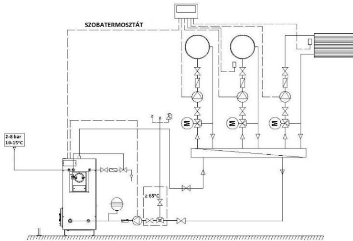
PHOENIX DUO csatlakoztatása háromutas szeleppel
